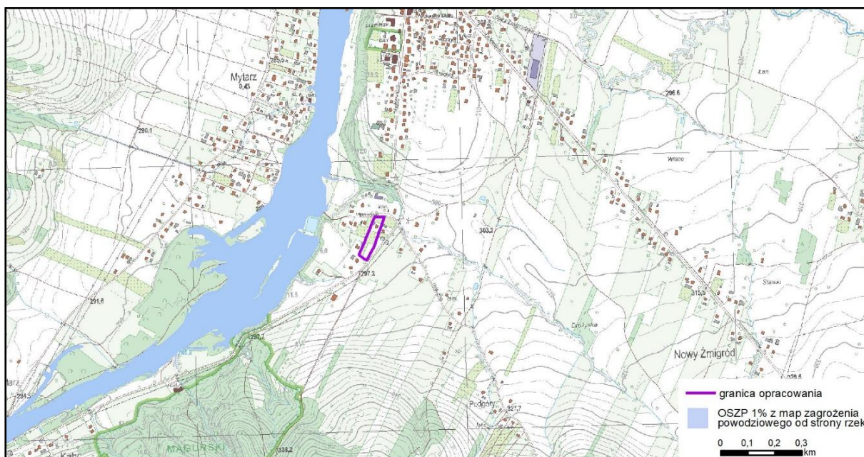
Ryc. 9. Lokalizacja analizowanego terenu na tle obszarów zagrożenia powodzią.
