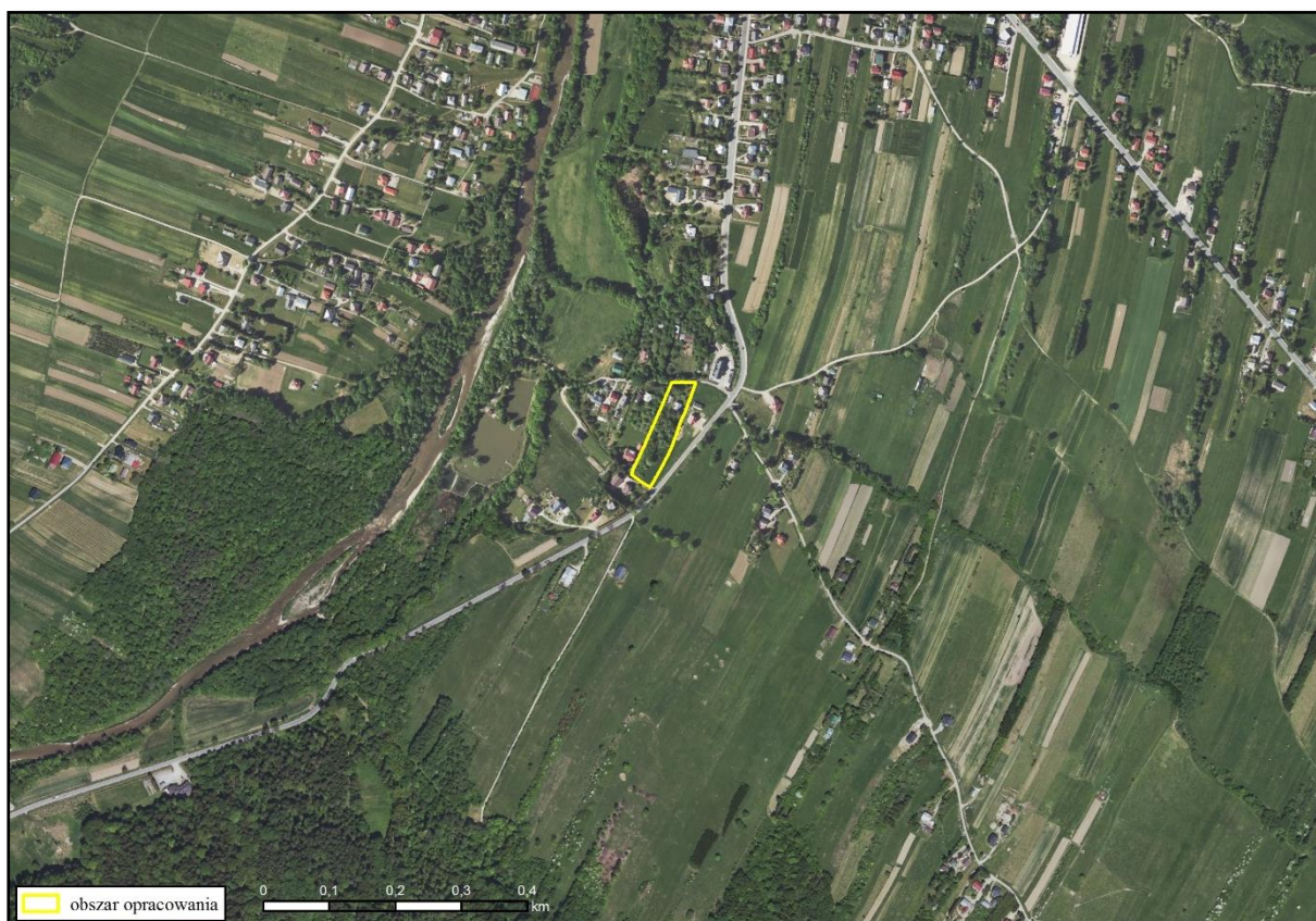
Ryc. 4. Lokalizacja analizowanego terenu na tle ortofotomapy.
