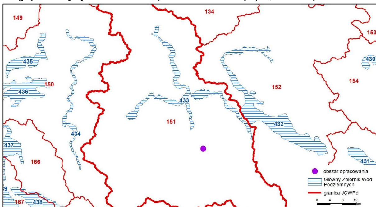
Ryc. 10. Położenie analizowanego terenu względem JCWPd i GZWP.
