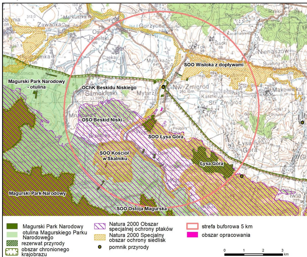
Ryc. 12. Obszary chronione w promieniu 5 km od obszaru opracowania.
