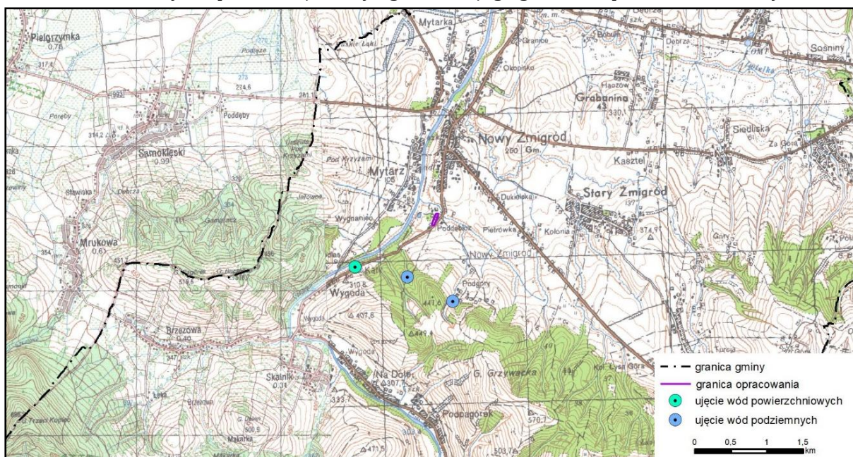
Ryc. 11. Ujęcia wód w gminie Nowy Żmigród.
