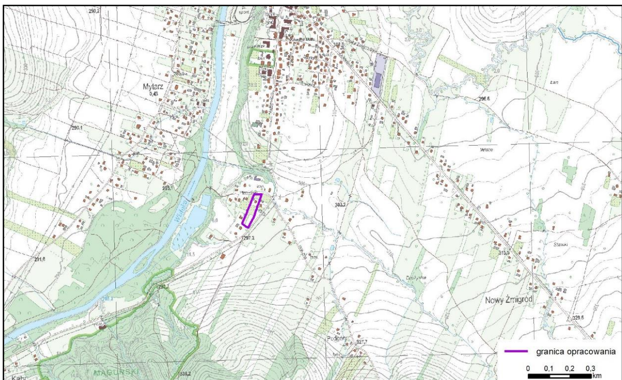
Ryc. 3. Lokalizacja analizowanego terenu na tle mapy topograficznej (2).
